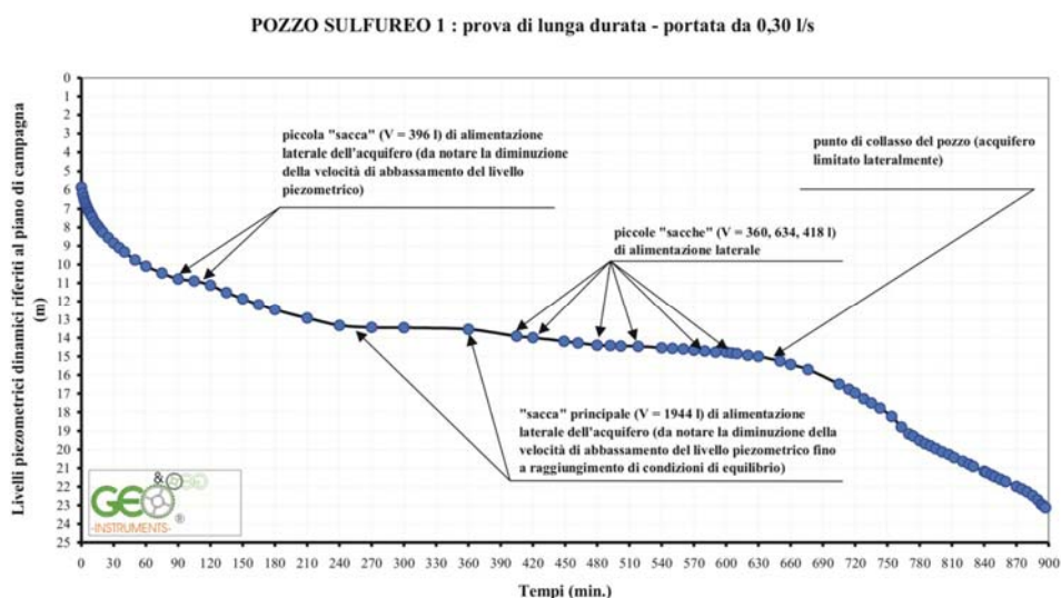
Fig. 3 – pozzo “Sulfureo 1” - abbassamenti piezometrici in funzione del tempo di pompaggio (LP → t) relativi alla prova di lunga durata; la curva mostra chiaramente la posizione delle sacche di alimentazione laterale dell’acquifero e il punto di inizio del collasso del pozzo
